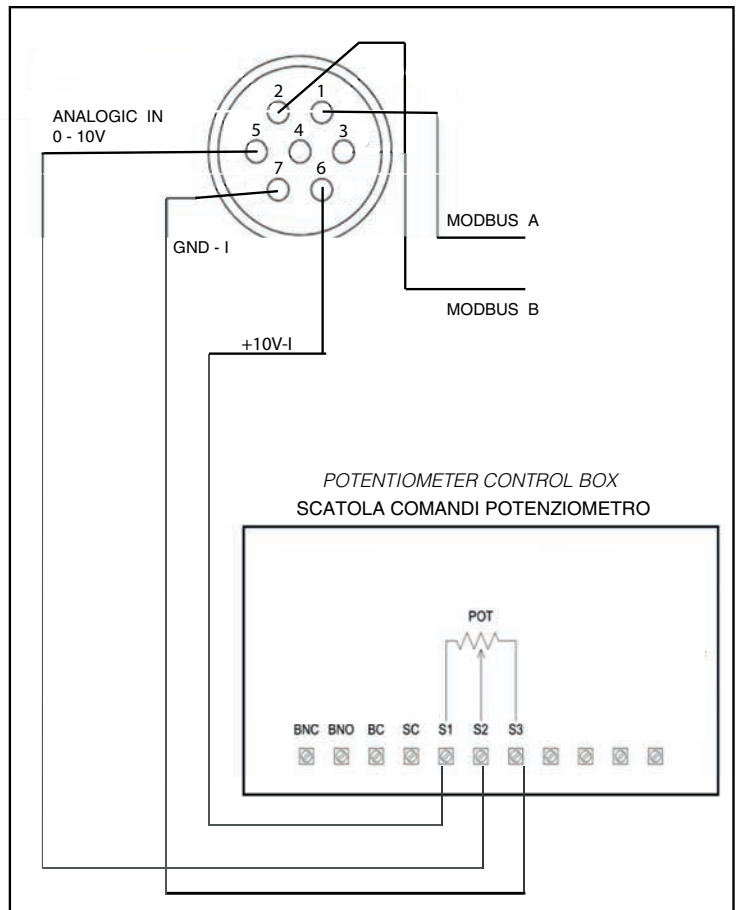
DETTAGLIO CONNESSIONI
