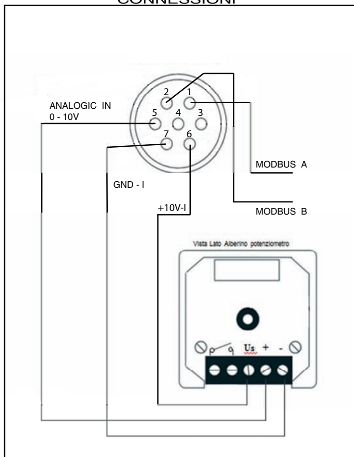
DETTAGLIO CONNESSIONI
