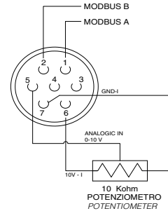
DETTAGLIO CONNESSIONI
